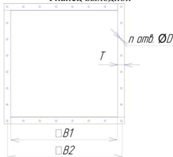
Фланец выходной
